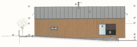
POHĽAD BOČNÝ - SEVEROZÁPADNÝ
