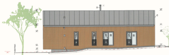
POHĽAD BOČNÝ - JUHOVÝCHODNÝ
